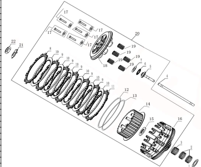
离合器总成 CLUTCH ASSY
