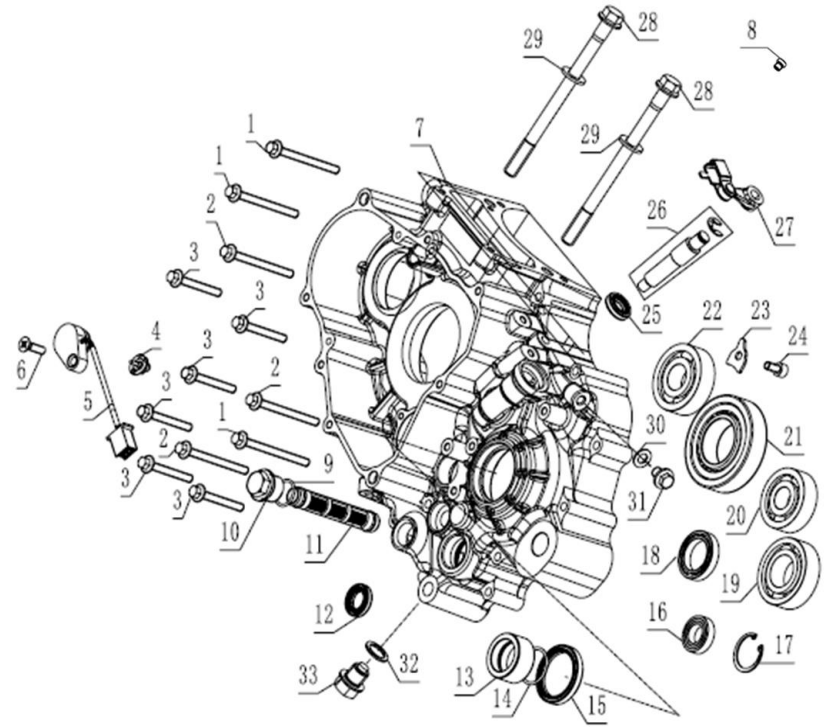
左曲轴箱 LEFT CRANKCASE
